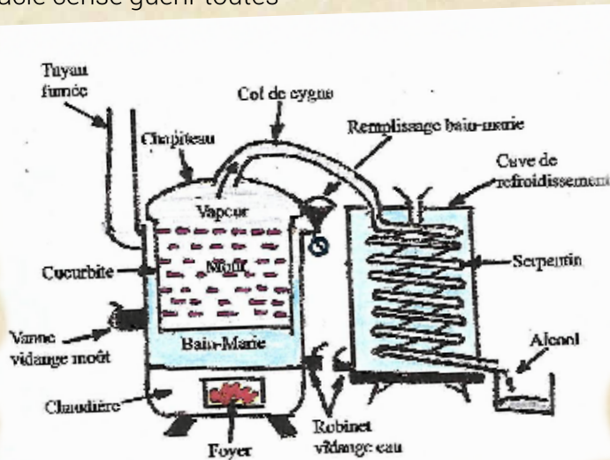
Schéma de fonctionnement d'un alambic
